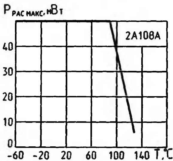
Зависимость предельной рассеиваемой мощности от температуры
