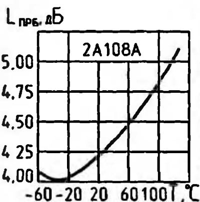
Зависимость потерь преобразования от температуры
