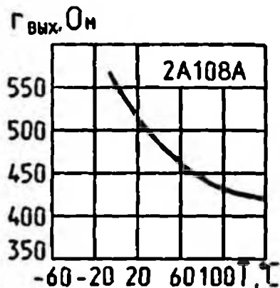
Зависимость выходного сопротивления от температуры
