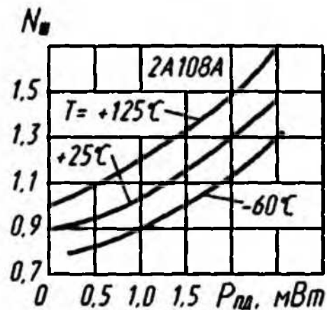
Зависимости выходного шумового отношения от непрерывной падающей СВЧ мощности
