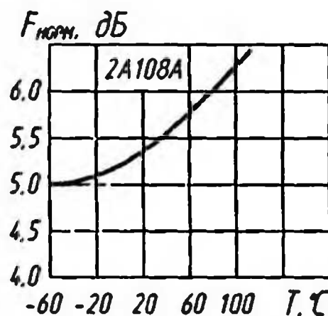
Зависимость нормированного коэффициента шума от температуры
