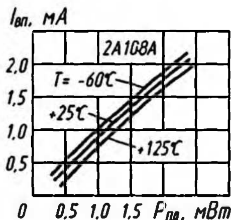
Зависимости выпрямленного тока от непрерывной падающей СВЧ мощности
