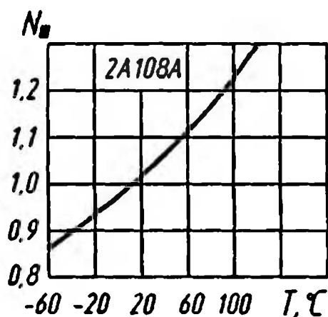
Зависимость выходного шумового отношения от температуры
