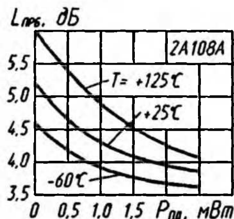
Зависимости потерь преобразования от непрерывной падающей СВЧ мощности
