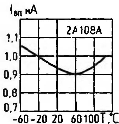
Зависимость выпрямленного тока от температуры
