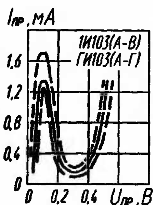
Зона возможных положений вольт-амперной характеристики
