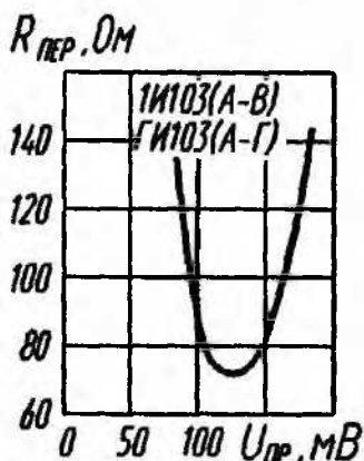
Зависимость отрицательного сопротивления перехода от напряжения
