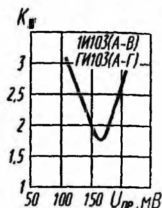
Зависимость коэффициента шума от напряжения
