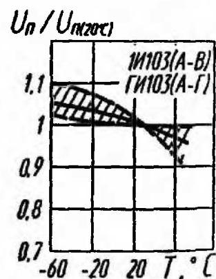
Зона возможных положений зависимости напряжения пика от температуры
