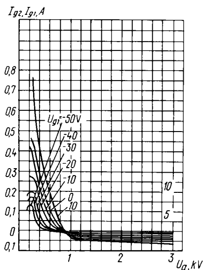
Усредненные сеточно-анодные характеристики: U_1 = 27 \text{ В} ; U_{g2} = 300 \text{ В} ; — — — — — ток сетки второй; — — — — — ток сетки первой Averaged Grid-Anode Characteristic Curves: U_1 = 27 \text{ В} ; U_{g2} = 300 \text{ В} ; — — — — — I_{g2} ; — — — — — I_{g1}
