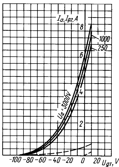
Усредненные характеристики: U_1 = 27 \text{ В} ; U_{g2} = 300 \text{ В} ; — — — — — анодно-сеточные; — — — — — сеточные (по сетке второй); — — — — — сеточные (по сетке первой) Averaged Characteristic Curves: U_1 = 27 \text{ В} ; U_{g2} = 300 \text{ В} ; — — — — — anode grid; — — — — — grid 2; — — — — — grid 1
